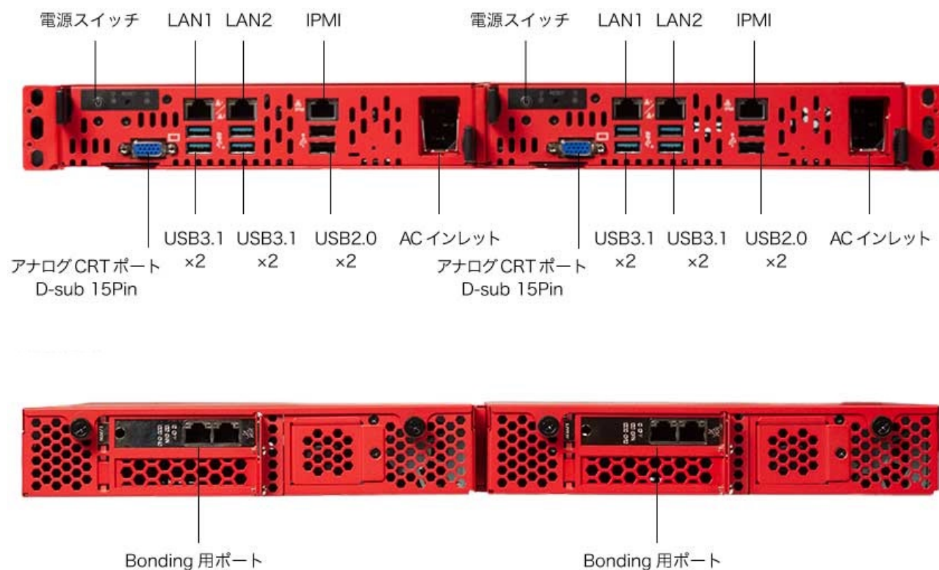
図1-2 フロントパネル
