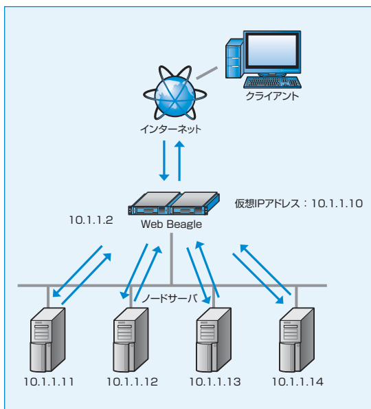
図2-2 透過型のネットワーク構成
